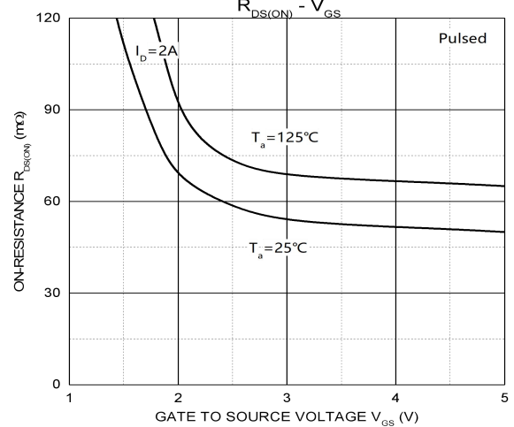
R_{DS(ON)} - V_{GS}
