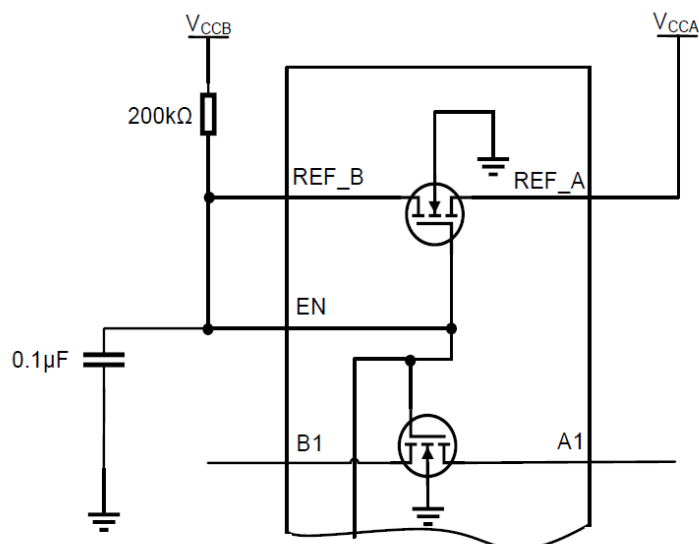
图 1. 直接将 EN 连接到 REF_B 并通过偏置电阻器连接到 V CCB
