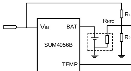
Figure 6. 电池充电温度设置
