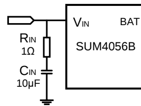
Figure 5. 提高热插拔可靠性
