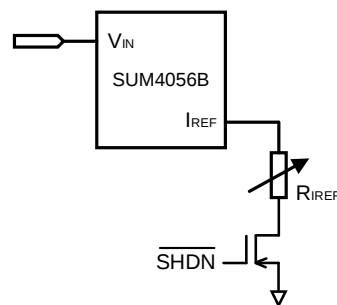
Figure 2. 充电电流设置 2
