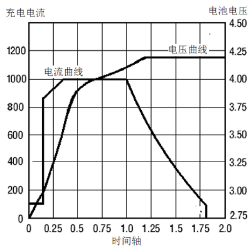
Figure 7. 三段式充电标准
