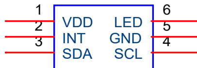
图1 引脚描述
