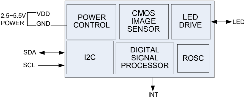
图2 功能框图
