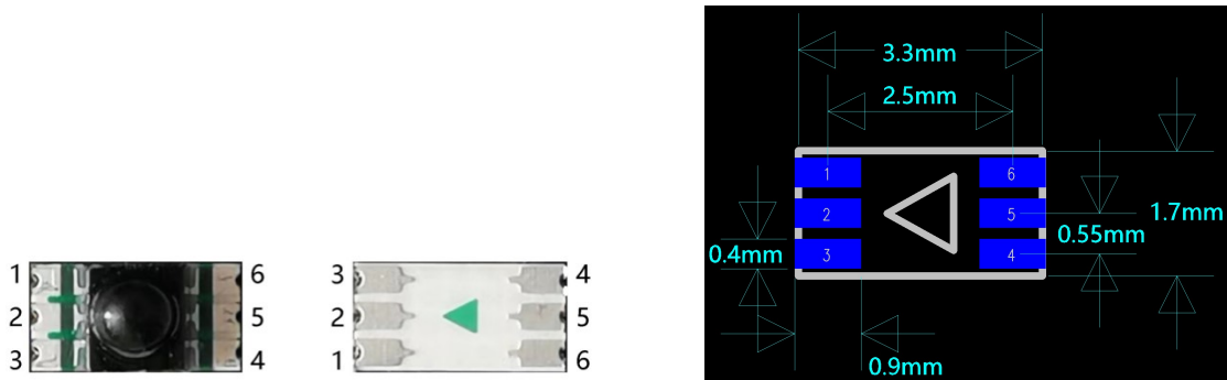
图7 SUMU002C PCB Layout尺寸参数 (外形尺寸3.3x1.7x2.0mm)
